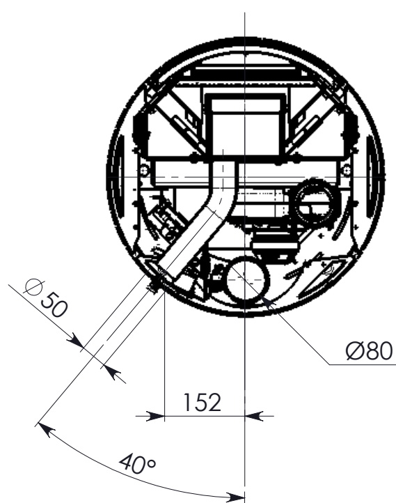
SEZIONE A-A SCALA 1 : 10
